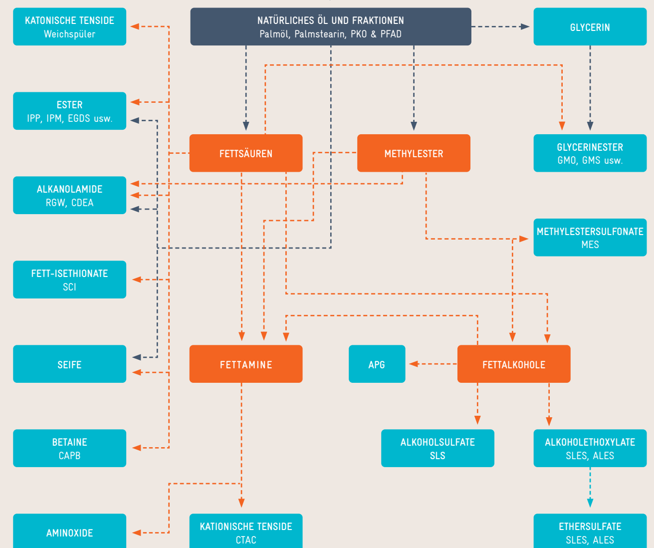
GRAFIK 2 Flowchart Produktionsschritte
